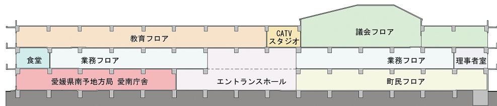
略断面図
